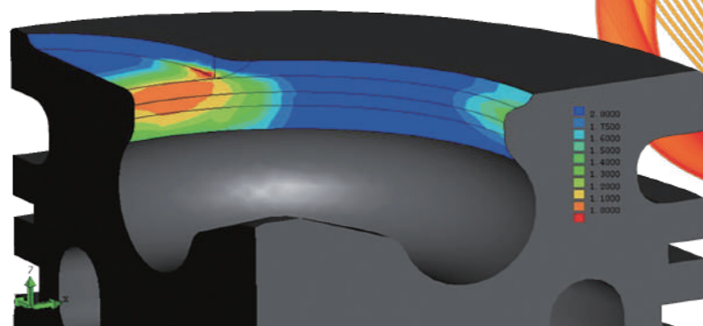
自動車用エンジンのピストン強度 (構造解析)
