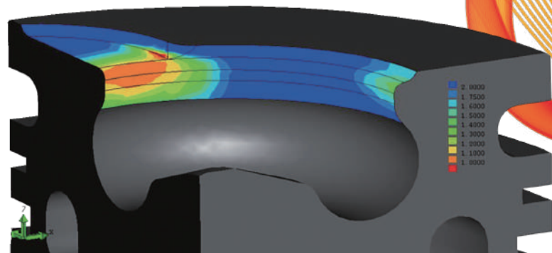
自動車用エンジンのピストン強度 (構造解析)
